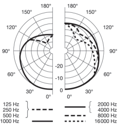
Diagramme polaire
