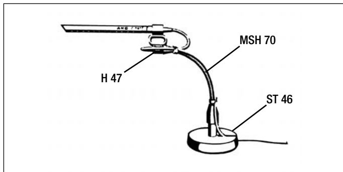
Fig. 6: Microfone montado num tripé de mesa
