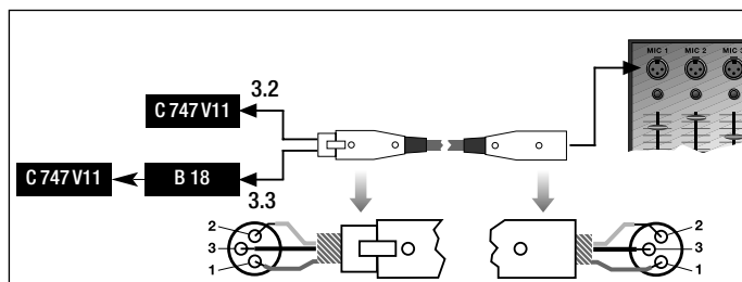
Fig. 1: Conexão numa entrada balanceada
