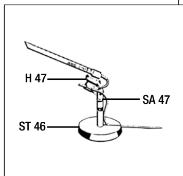
◀ Fig. 8 : Fixation directe du microphone sur un support de table
