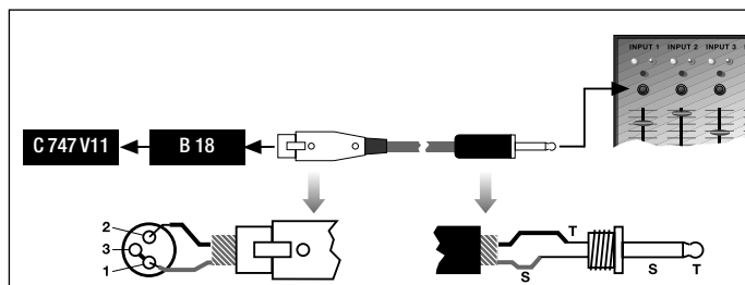
Fig. 2: Conexão numa entrada desbalanceada
