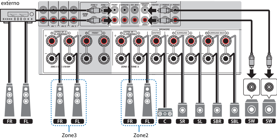
Amplificador de potencia externo
