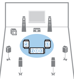
Medición múltiple (5 posiciones de escucha)
