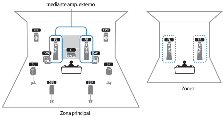
Amplificador de potencia externo
