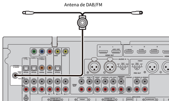
La unidad (parte trasera)
