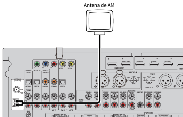
La unidad (parte trasera)
