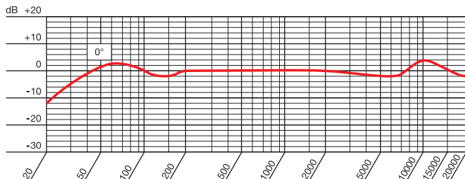
Frequenzkurve
