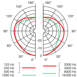
Polardiagramm
