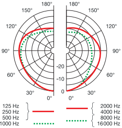
Diagrama polar
