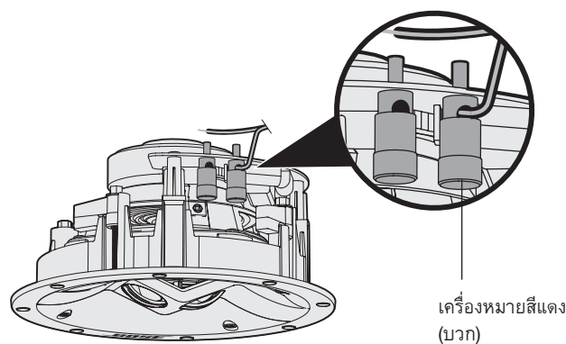
ลำโพง Virtually Invisible® 591
