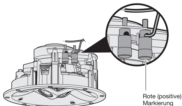
Virtually Invisible® 591 Lautsprecher
