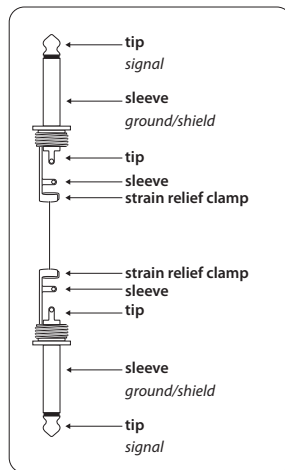
Fig. 4.1: Cable con conectores jack mono de 6,3 mm
