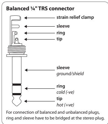
Fig. 4.2: Jack estéreo
