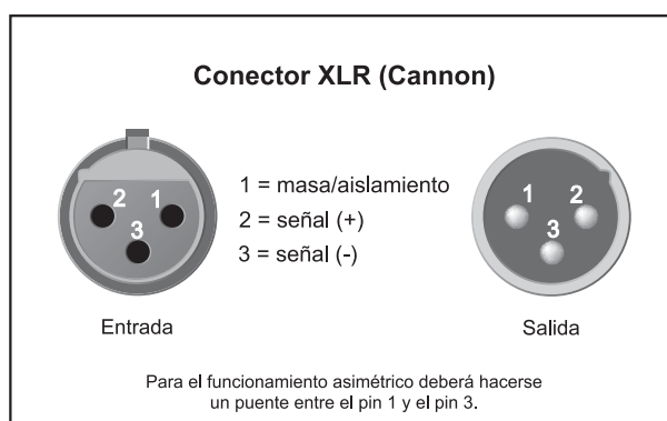
Fig. 3.1. Conexión XLR
