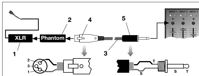
Fig. 2 : Raccordement sur une entrée asymétrique
