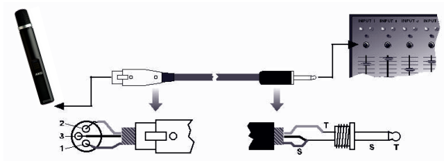
Figura 4: Collegamento tramite cavo simmetrico
