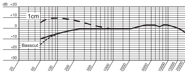
Frequenzgang (Niere)
