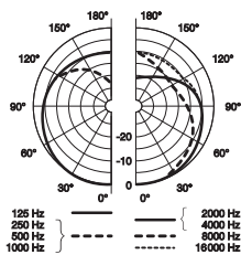
Diagramme polaire (hypercardioïde)
