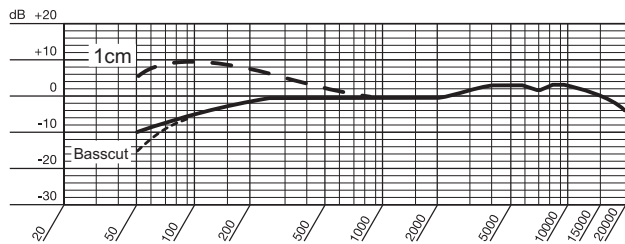
Respuesta de frecuencia (cardioide)
