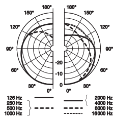
Polardiagramm (Hyperniere)
