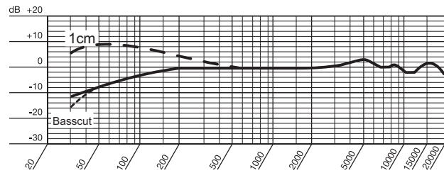
Respuesta de frecuencia (hipercardioide)
