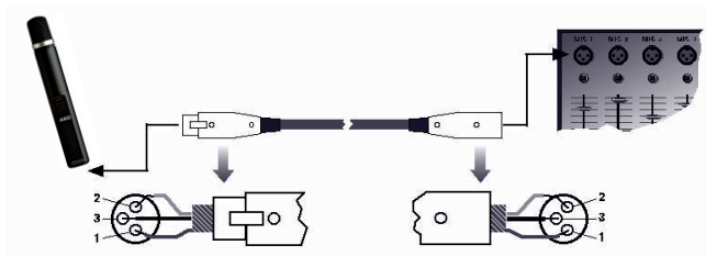
Figura 5: Collegamento tramite cavo XLR simmetrico
