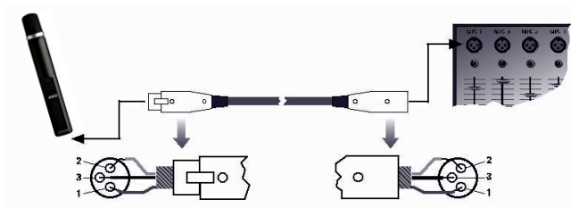
Figura 3: Collegamento tramite cavo XLR simmetrico
