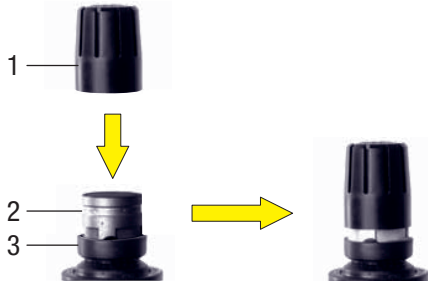
Abbildung 6: PPC1000/PB1000 montieren
