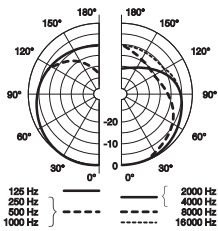
Diagramma polare (ipercardioid)
