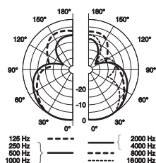
Diagrama polar (hipercardióide)
