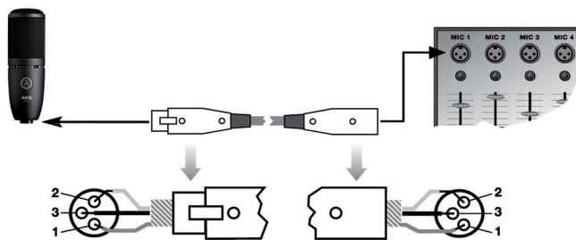
Figure 2: Connexion sur une entrée symétrique avec alimentation fantôme
