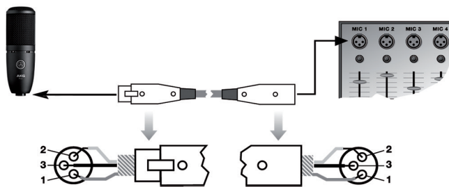
Figura 2: Conexión a una entrada equilibrada con potencia fantasma
