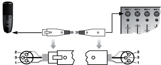
Abbildung 2: Anschluss an einen symmetrischen Eingang mit Phantomspeisung
