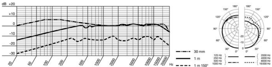
Réponse en fréquence et diagramme polaire pour HSC 171, HSC 271
